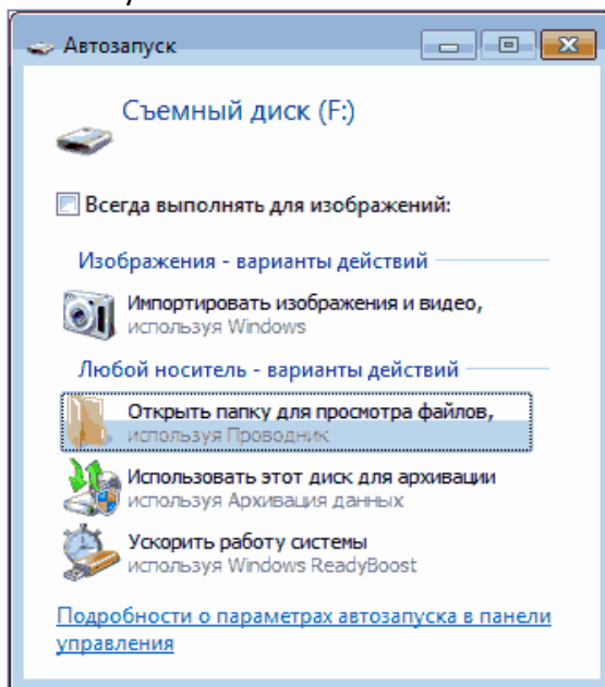
Рисунок 1 Диалог "Автозапуск"
