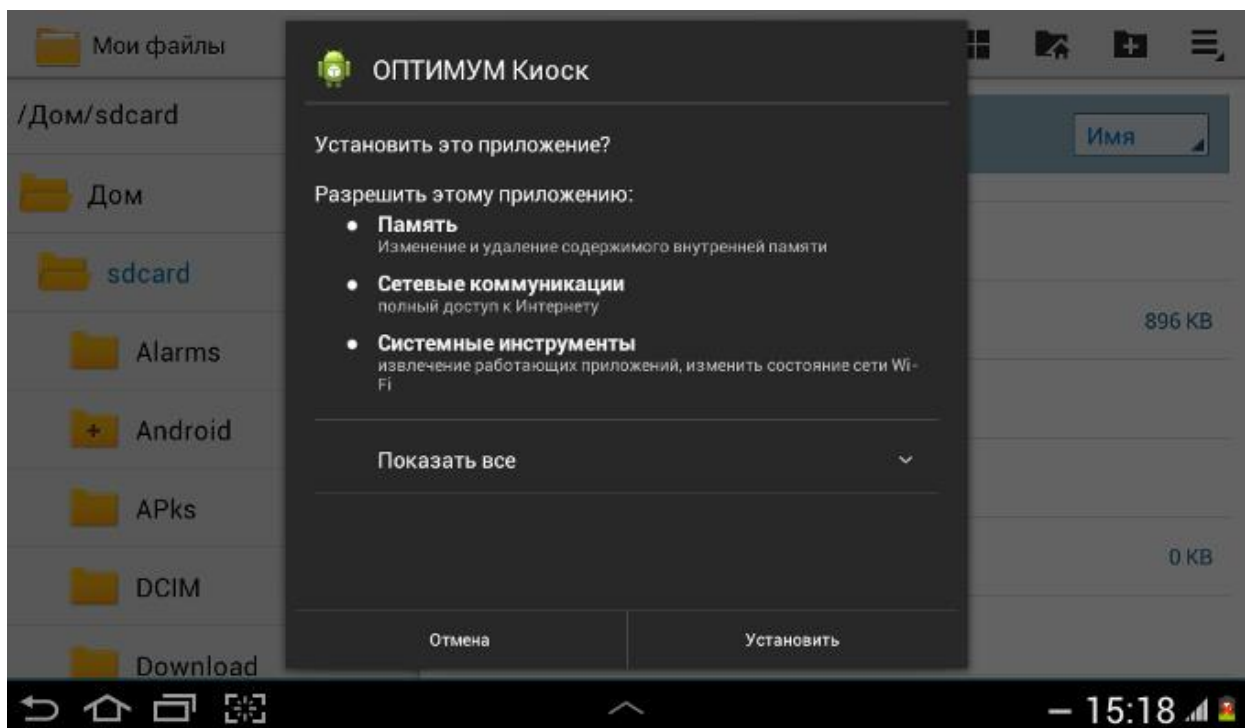
Рис 3. Окно подтверждения установки приложения
